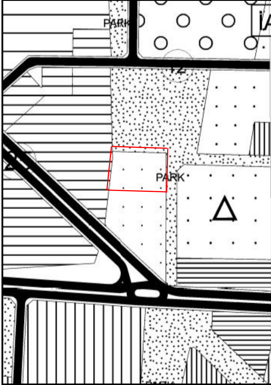
Şekil 2:Mer'i Nazım İmar Planı
